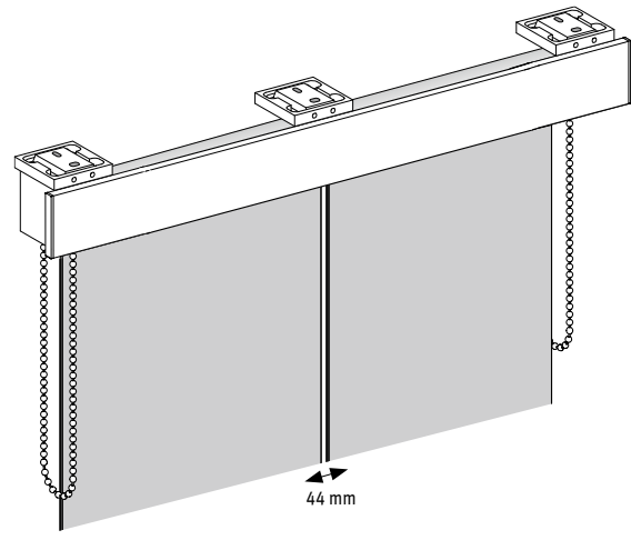
Deckenmontage
