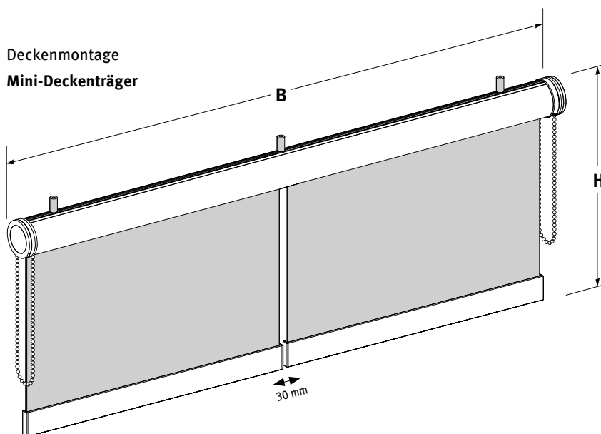
Deckenmontage Mini-Deckenträger Click
