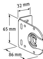
Metall-Zwischenträger PH4001-012 silber
