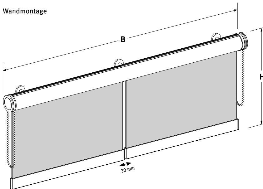
Deckenmontage Mini-Deckenträger
