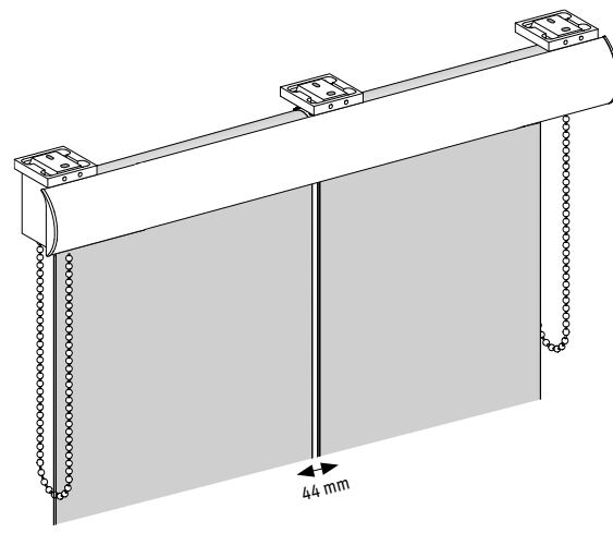
Deckenmontage
