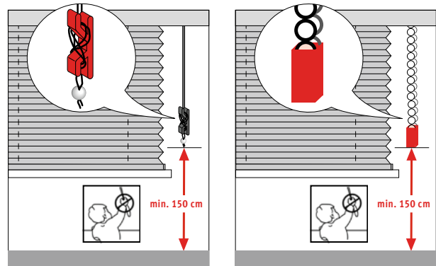
Schnurwickelsystem für Bedienvariante mit Schnurzug.
