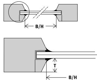
Schräges Profil
