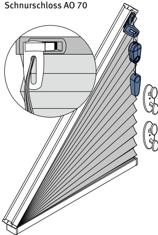
Detailabbildung Schnurschloss AO 70
