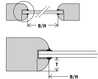
Rundes Profil
