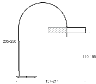
Bogenleuchte / Arc lamp BW-L-101-400
